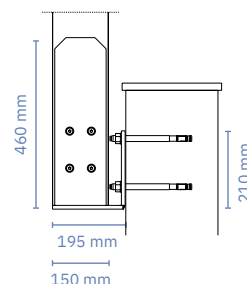
Säulen 150/150
