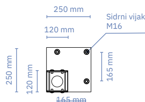
Säulen 120/120
